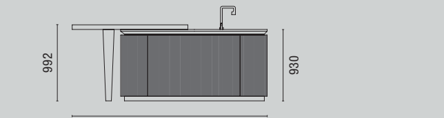
PROSPETTO G-G Front view G-G
