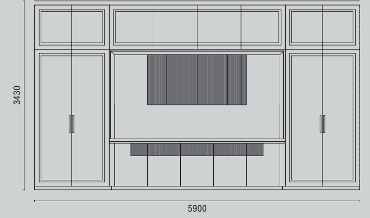
PROSPETTO B-B Front view B-B
