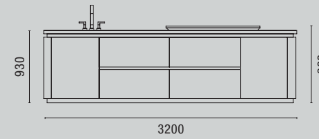
PROSPETTO C-C Front view C-C
