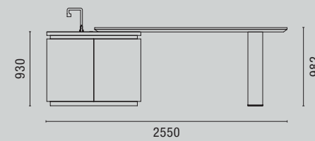
PROSPETTO E-E Front view E-E
