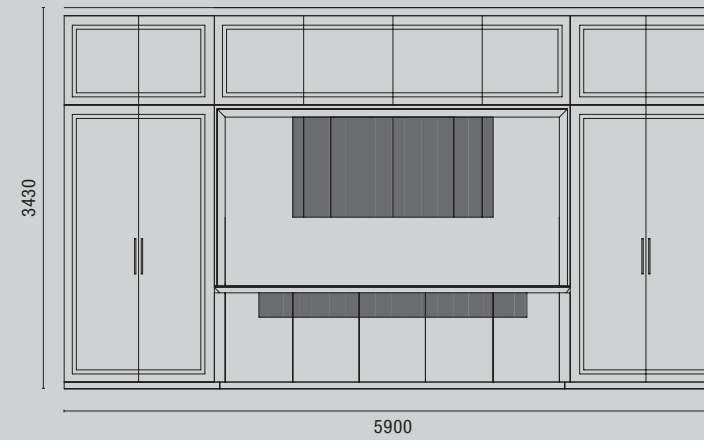
PROSPETTO C-C Front view C-C
