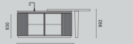
PROSPETTO F-F Front view F-F
