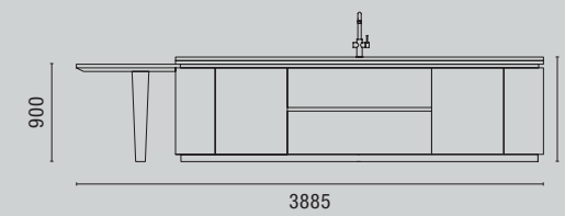
PROSPETTO E-E Front view E-E
