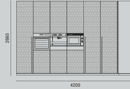
PROSPETTO A-A Front view A-A
