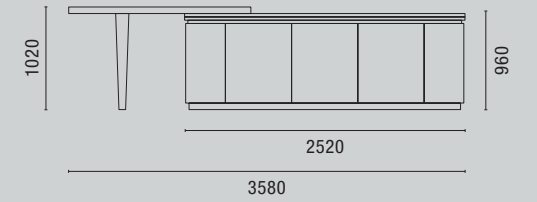
PROSPETTO F-F Front view F-F
