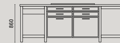
PROSPETTO B-B Front view B-B
