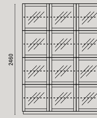
PROSPETTO D-D Front view D-D
