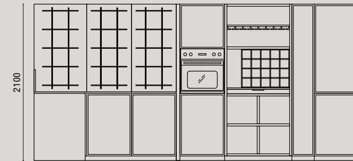
PROSPETTO C-C Front view C-C
