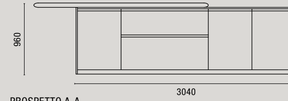
PROSPETTO A-A Front view A-A
