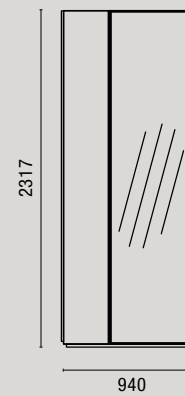
PROSPETTO E-E Front view E-E
