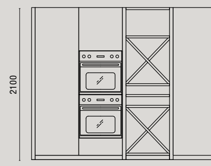
PROSPETTO E-E Front view E-E
