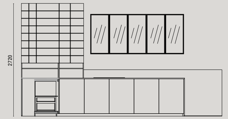
PROSPETTO B-B Front view B-B
