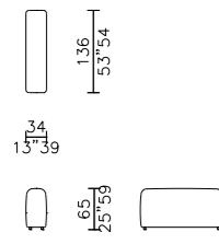
schienale - backrest 136
