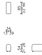
bracciolo - armrest 85
