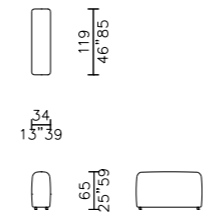
schienale - backrest 119
