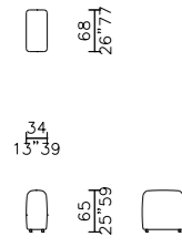
schienale - backrest 68
