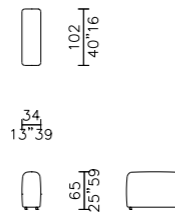
schienale - backrest 102
