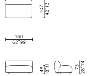
elemento - unit 160
