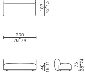
elemento - unit 200
