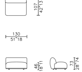
elemento - unit 130
